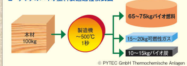
ピーテックのバイオ燃料製造過程模式図
